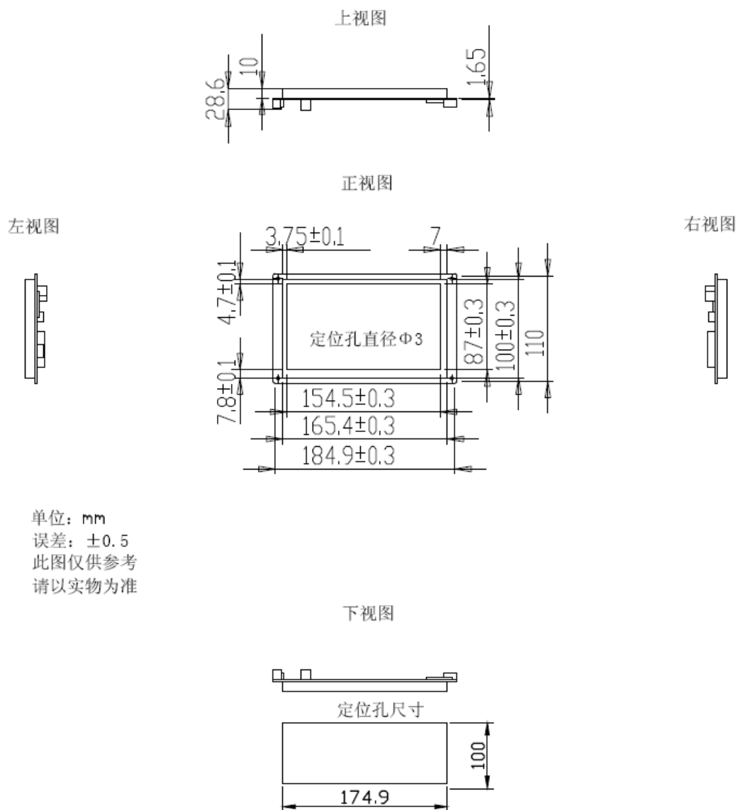
◆ LJD-eWinV5-EK7 尺寸图: 单位 mm
