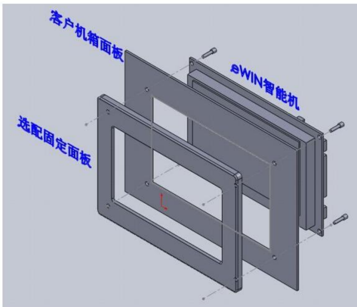
LJD-eWinV5-EK7 安装示意图:
